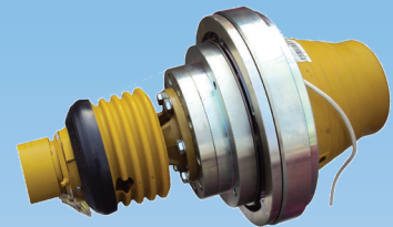
Elektromagnetkupplung
