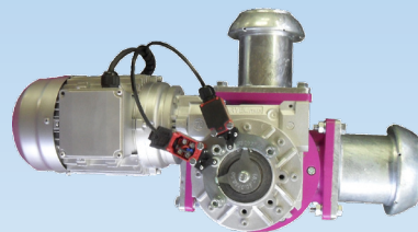
Dreiweghahnen für Umschaltung Wasser - Gülle per Funk
