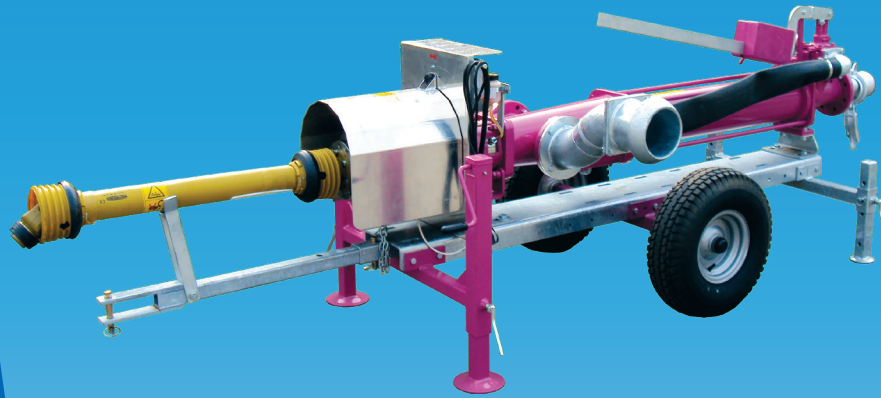
Pumpe mit 2-Rad Wagen, Elektromagnet- kupplung und Funksteu- erung AGROPILOT
